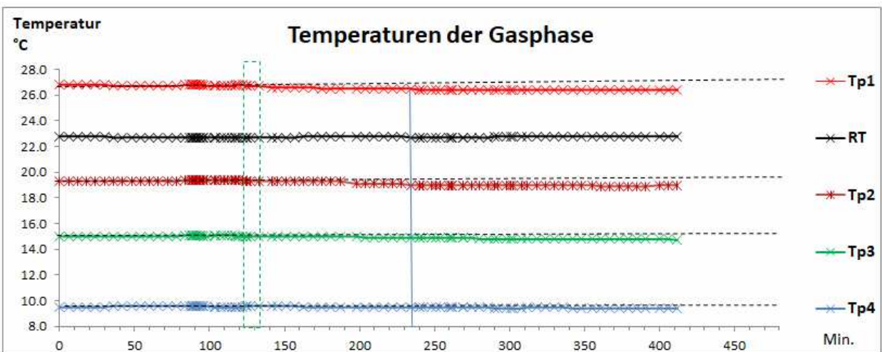
Abb. 7c: Freon-Isolations-Experiment: Temperatur-Daten der Messfühler.
