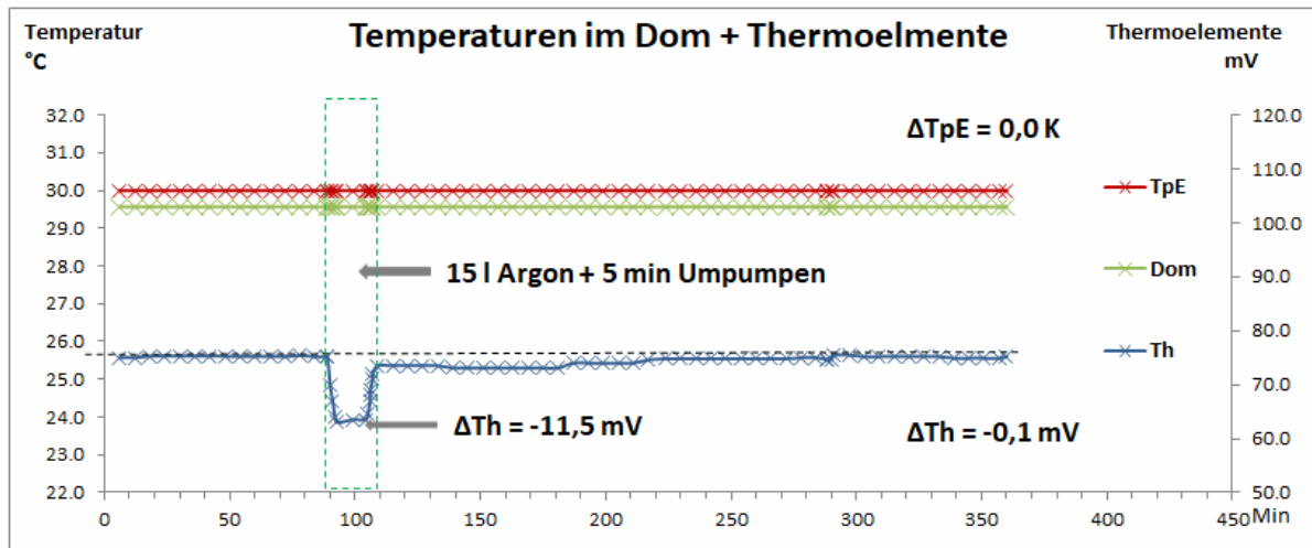
Abb. 5a: Argon-Kontrollexperiment Nr. 6: Endkonzentration 13 Vol.-% Argon
