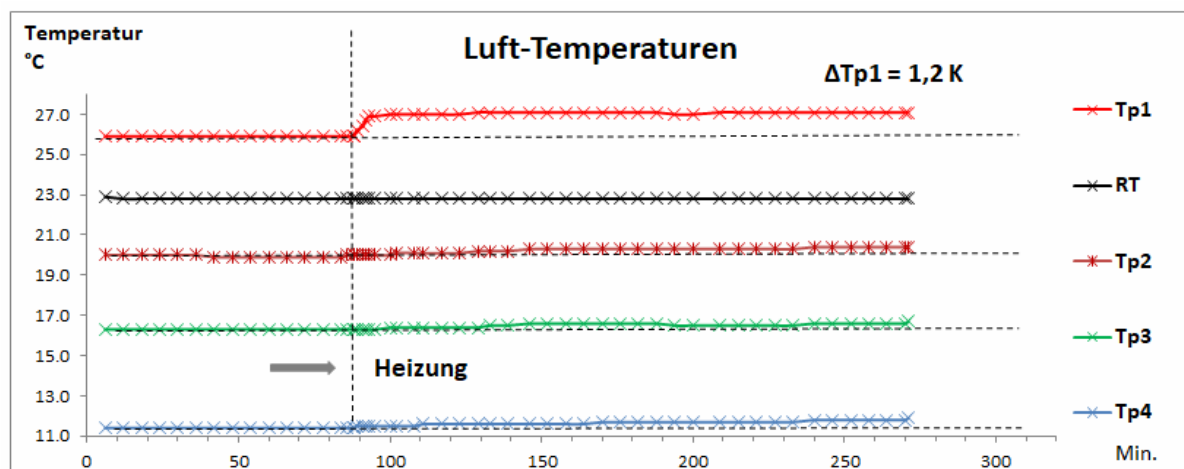
Abb. 8b: Veränderungen der Lufttemperatur beim Einschalten der Heizung
