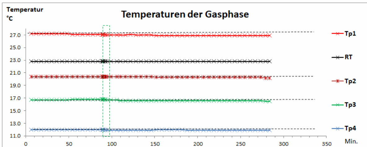
Abb. 4b: Freon-Experiment: Temperatur-Daten der Messfühler.
