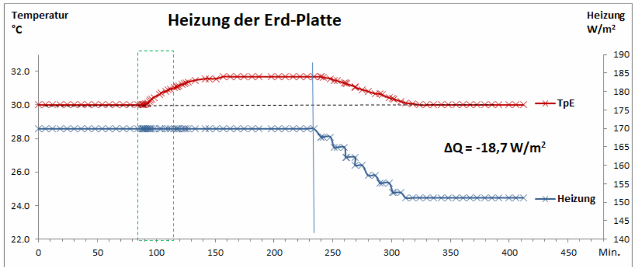
Abb. 7b: Nachweis des Isolations-Effektes von Freon 134a
