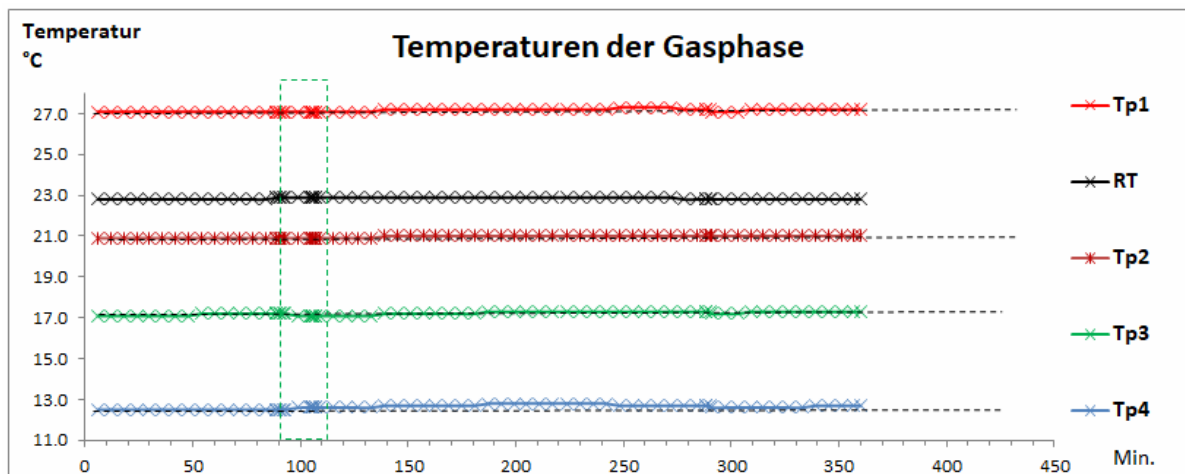
Abb. 5b: Argon-Kontrollexperiment: Temperatur-Daten der Messfühler.
