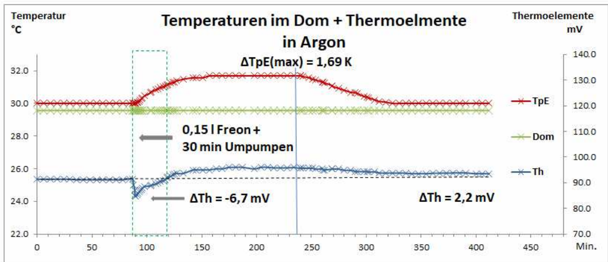
Abb. 7a: Freon-Experiment Nr. 15: Endkonzentration 0,13 Vol.-% Freon 134a
