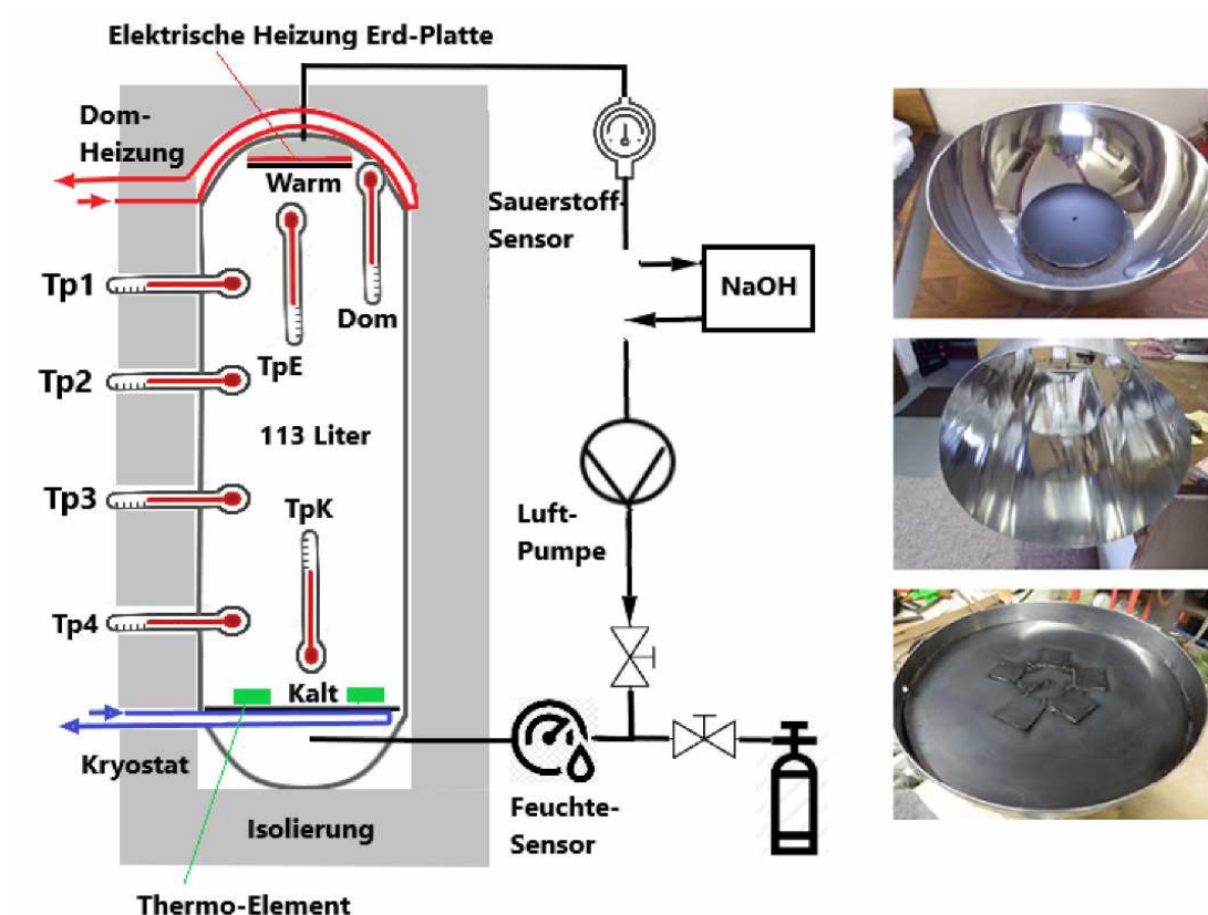
Abb. 1: Links: Schematischer Aufbau des Experimentes. Rechts: Erd-Platte im Dom, Verbindungsrohr und kalte Platte.
