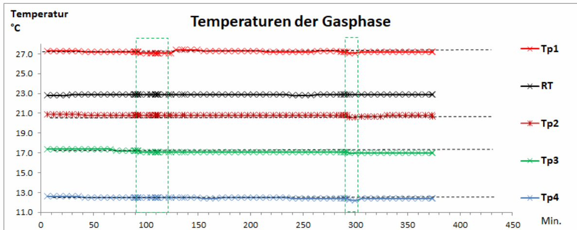
Abb. 2b: CO 2 -Experiment: Temperatur-Daten der Messfühler.
