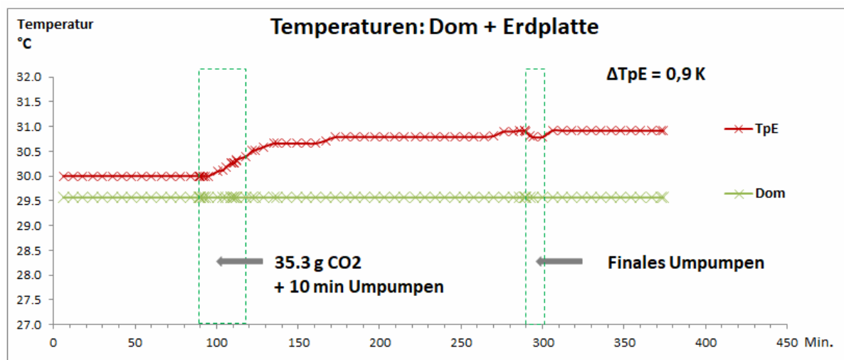
Abb. 2a: CO 2 -Experiment Nr. 30: Endkonzentration 15,4 Vol.-% CO 2
